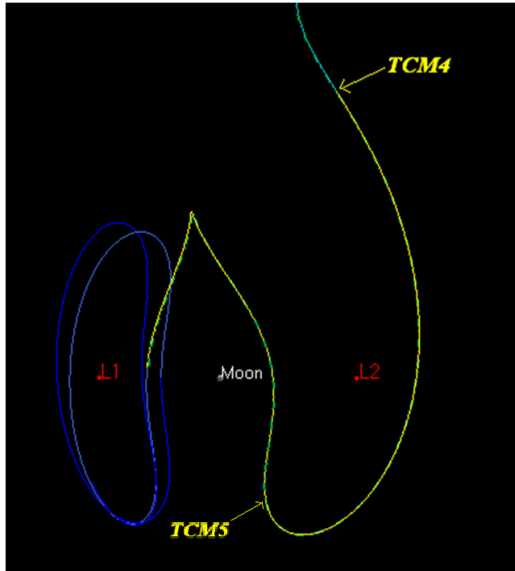
Figure 16. P2 TCM4/TCM5 Trajectory
